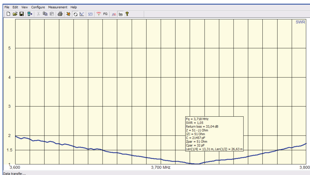
Mätning av SWR på min dipol. Kurvan visar värdet mellan 3.6 till 3.8 Mhz
