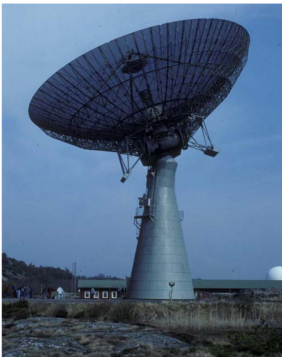
En jätteparabol, drygt 25 m i diameter. Råö rymdobservatorium, på Onsalahalvön.
